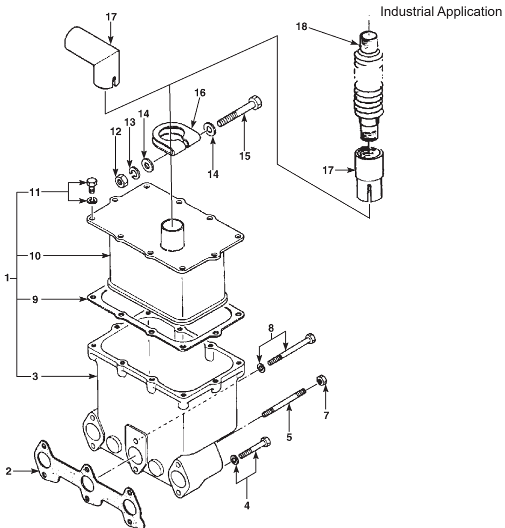
673 MUFFLER
